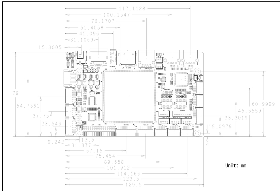
图 5.2-1 鲁班猫 1HS 底板正面机械尺寸图
