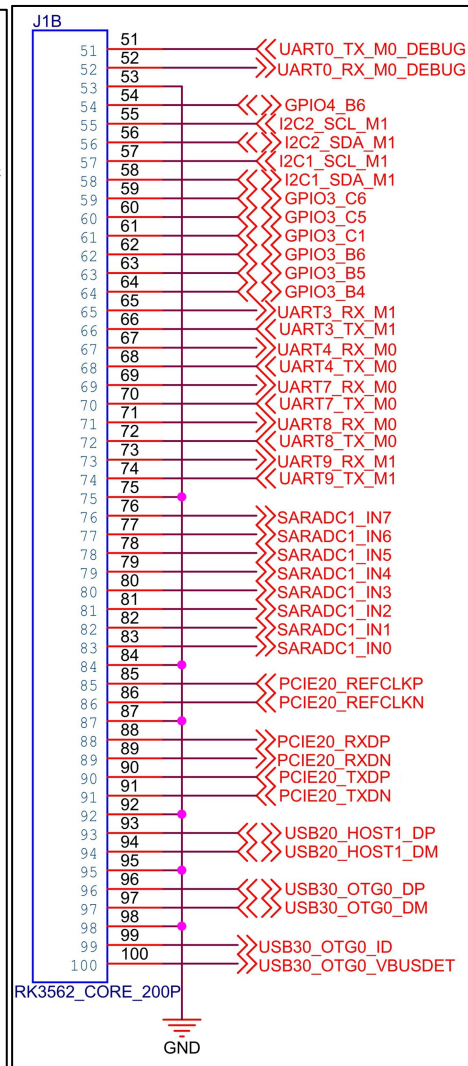
图 4.6-2 J1B 连接器原理图
