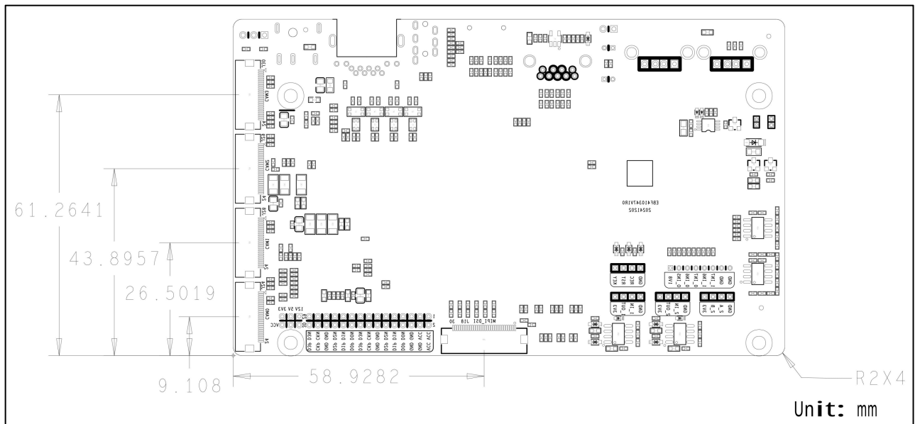
图 5.2-2 鲁班猫 1HS 底板背面机械尺寸图
